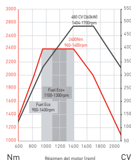
DE13 - 480 CV
